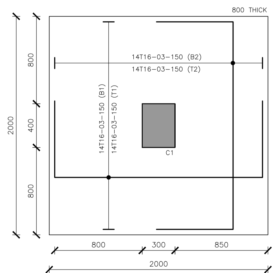
FOOTING F1
